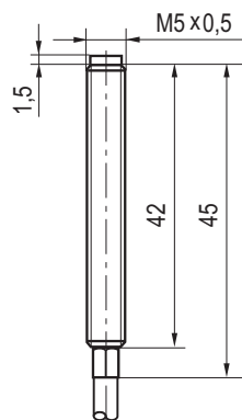
Габаритный чертеж
